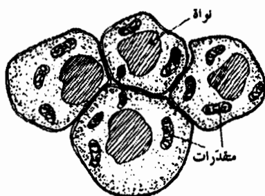
خلايا حيوانية
