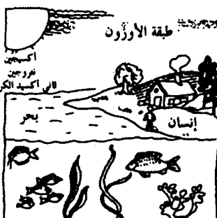
الأرض الحالية
