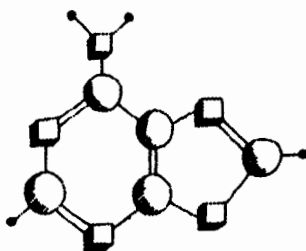
الأدينين
