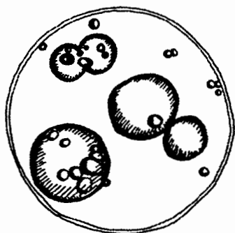
قطيرات من البروتينات المهيئة والمائلة للقوصرات
