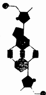
زوج غوانين-سيتوزين
