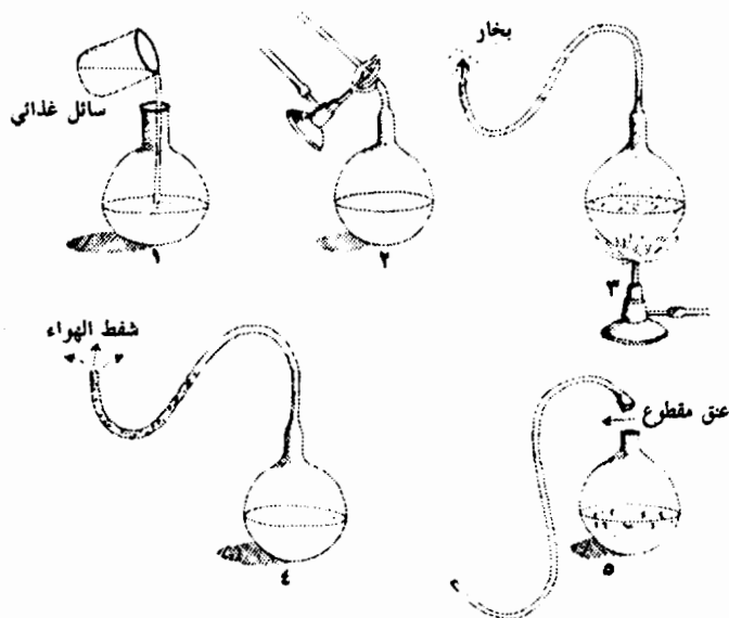
تجربة باستور
